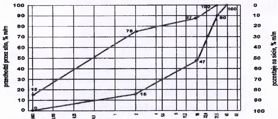
Rys. Krzywe graniczne uziarnienia mieszanki kruszywa niezwiązanego 0/31,5 mm do dożwirowania dróg gminnych.
